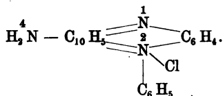
Rosindulin.
